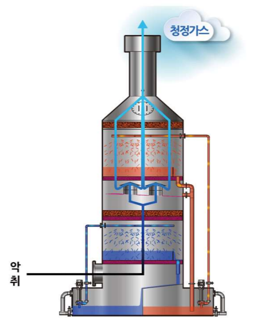
1탑 2단 약액탈취기
