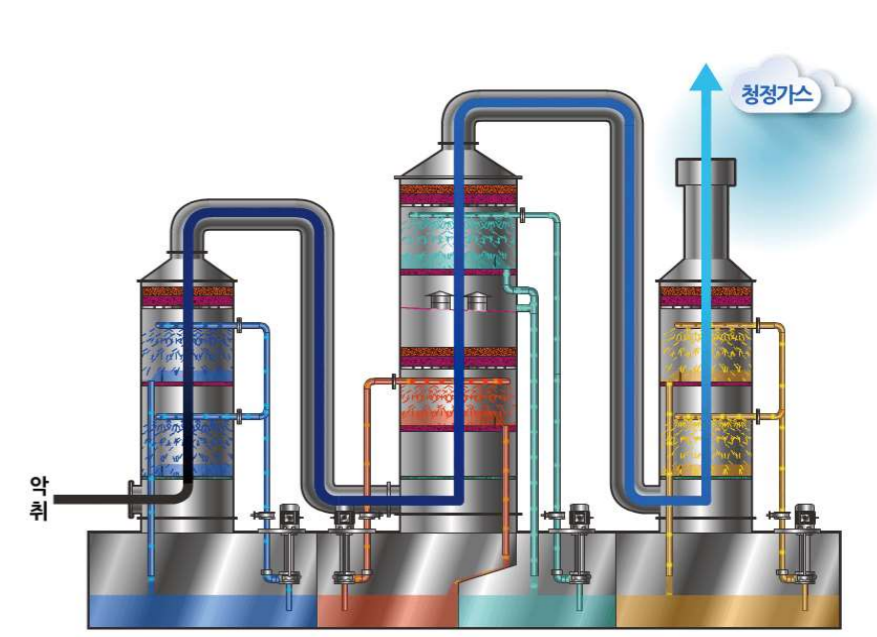
다탑 다단 약액탈취기
